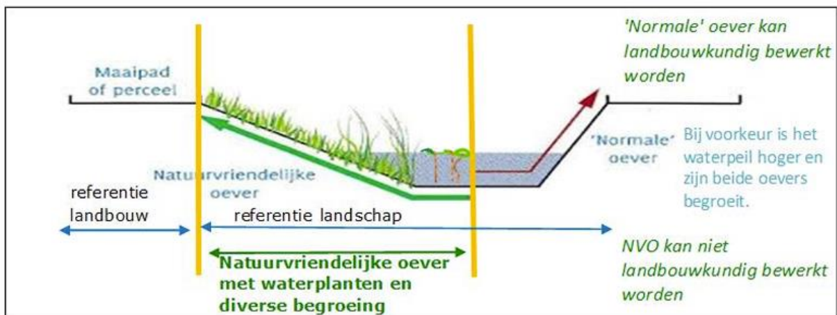
Figuur 1: Tekening natuurvriendelijke oever (NVO) © BoerenNatuur.
